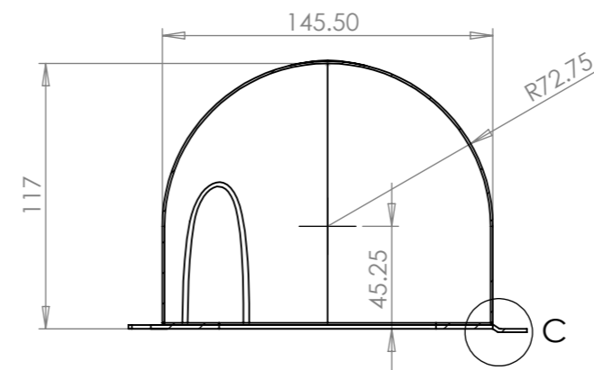
SECTION - SCALE 1 : 3
