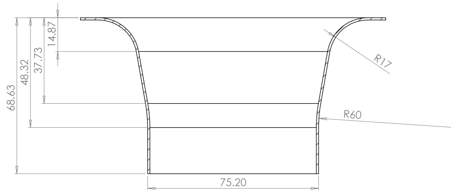
SECTION D-D SCALE 1 : 1
